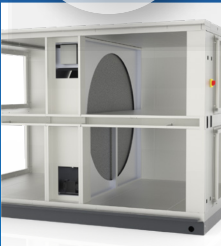
Récupérateur rotatif
